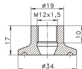
Adaptermuffe für TriClamp AMC-032
