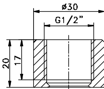
Zylindrische Einschweißmuffe EMZ-120
