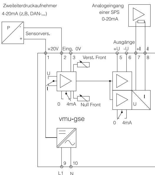
vmu-gse mit Anschluß eines Zweileitersensors
