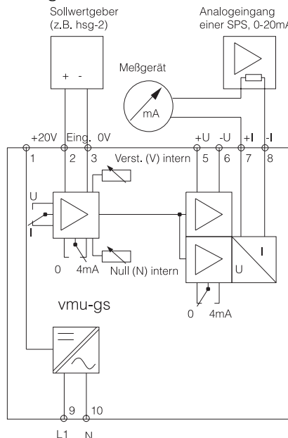
vmu-gs mit Anschlußschema für Abgleich
